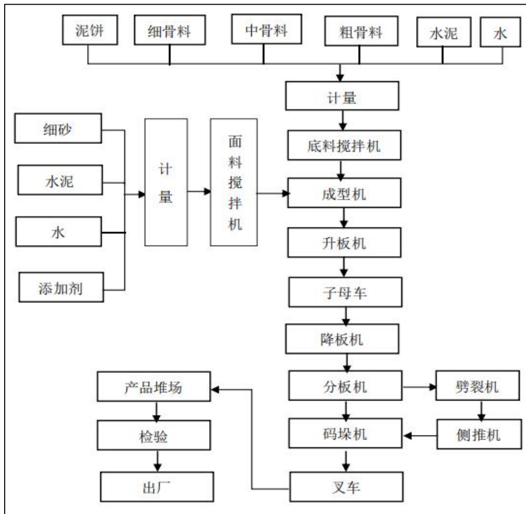
图3 一般固废综合利用生产线工艺流程图②
